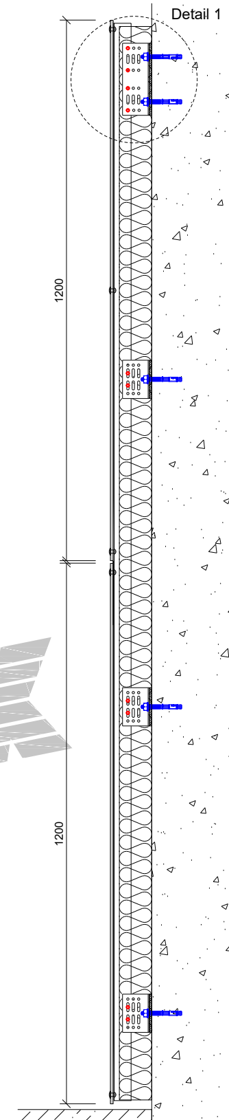
SECTION A-A SCALE 1:12
